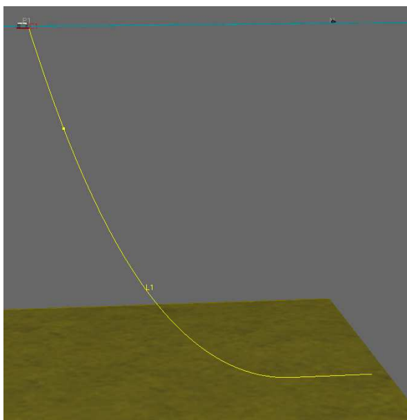
Figura 3. Modelagem de um riser de produção em catenária no programa ANFLEX
