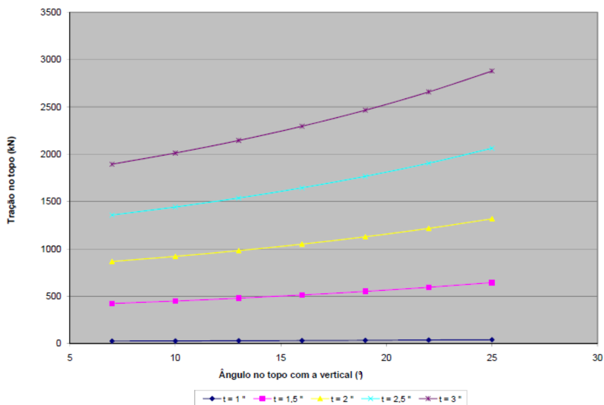
Fig. 5 – Curva de esforços gerada por modelagem de riser em RPCM a 3000 m de lâmina de água sob condições de ondas decenárias.
