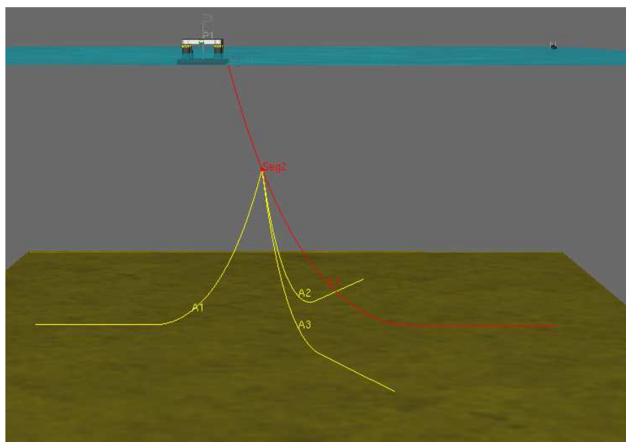
Figura 4. Modelagem de uma opção estabilizadora de um riser de produção em catenária feito de RPCM
