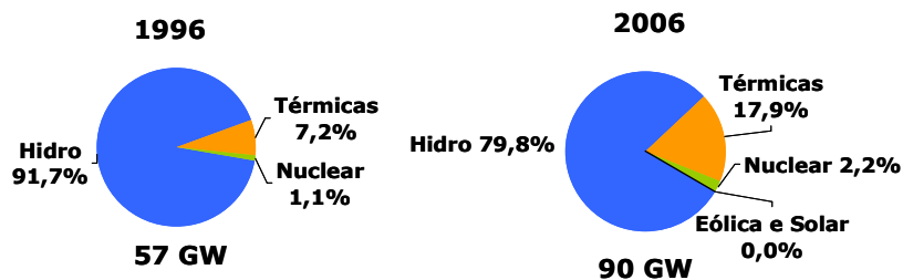
Figura 3 - Capacidade Instalada de Geração de Energia Elétrica no Brasil em 1996 e 2006 Fonte: Balanço Energético Nacional (BEN, 2006) para 1996 e www.aneel.com.br (ANEEL, 2007) para 2006
