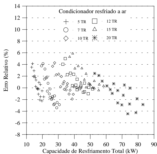
Figura 4 - Valores calculados pelo modelo de condicionador comparados aos de catálogo, em todas as condições de operação disponíveis.
