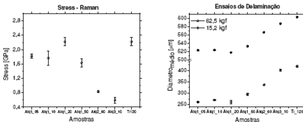
Figura 4. Resultados das medidas de stress e dos ensaios de delaminação nas ferramentas.
